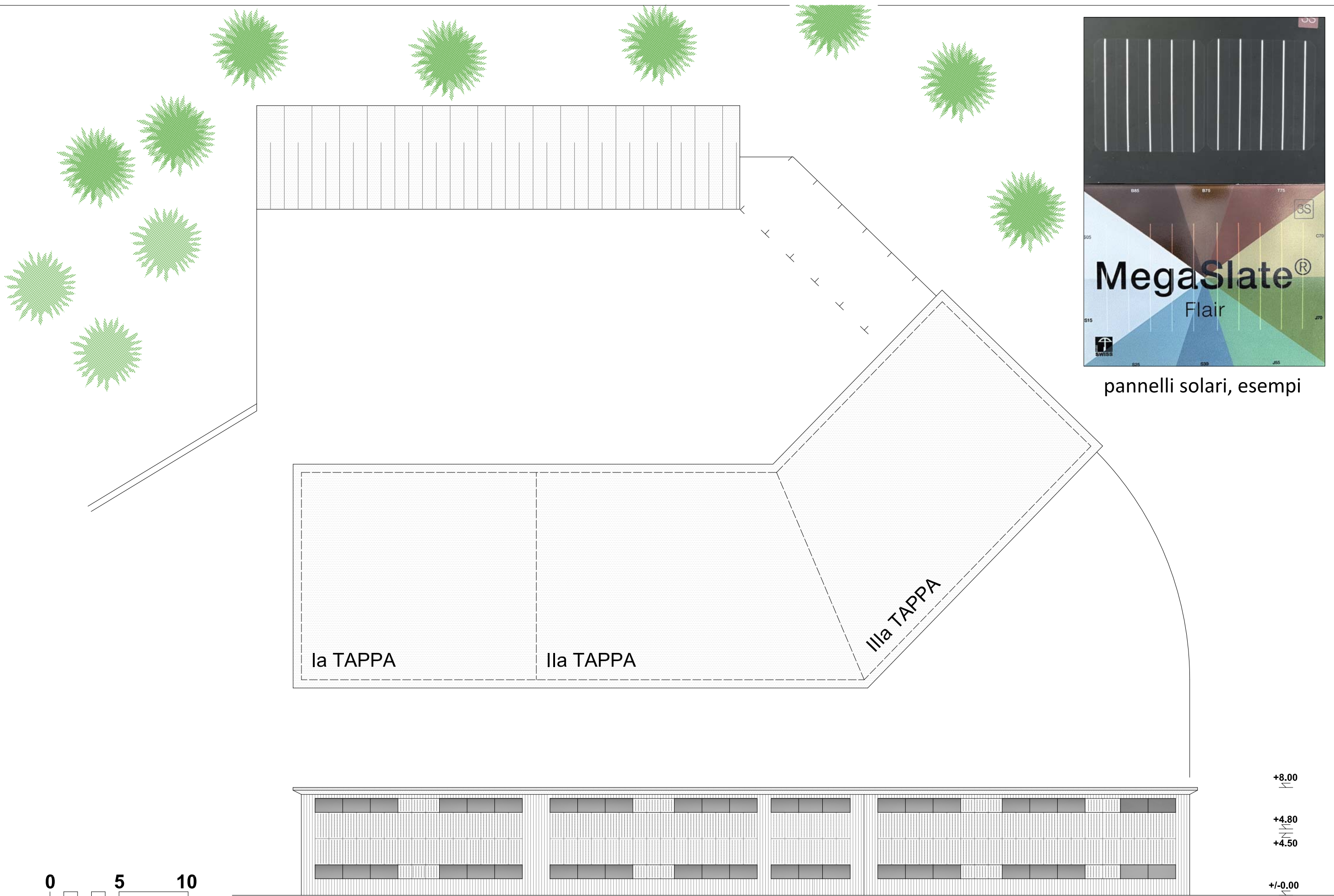
02, Pra d'Zura, strutturazione, schema facciate 1:250
