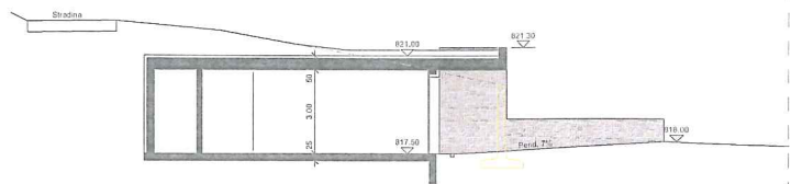
Sezione B - B
