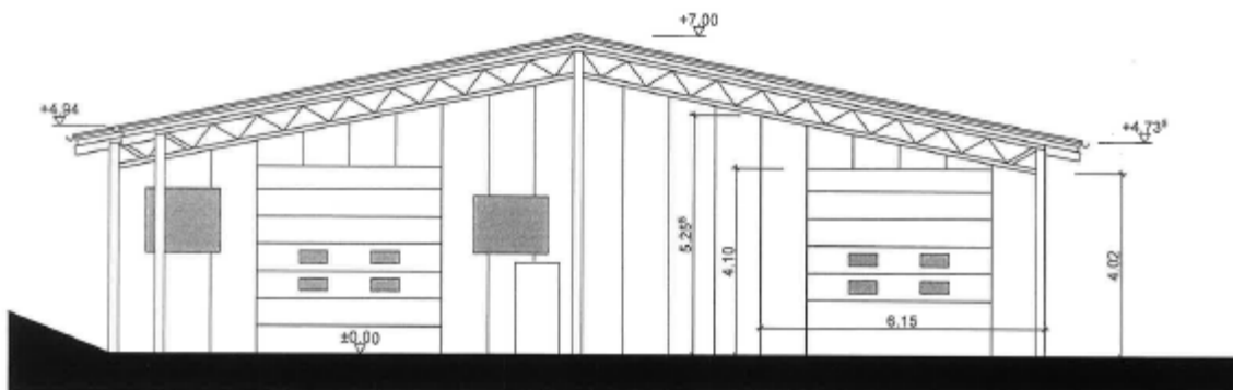
PROSPETTO OVEST S. 1:100
