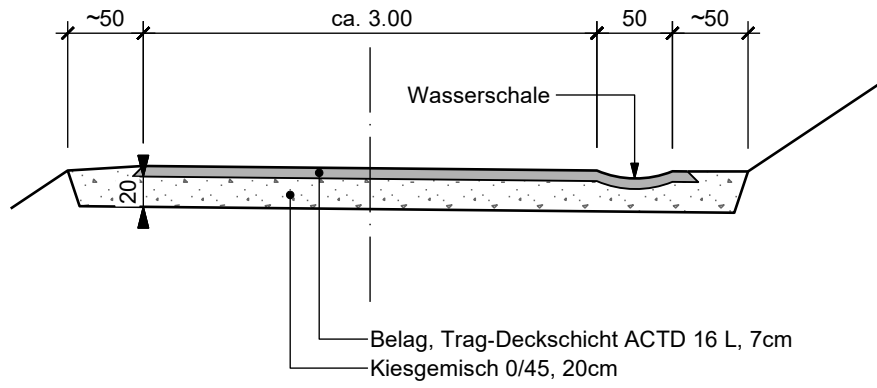
Normalprofil 1:50
