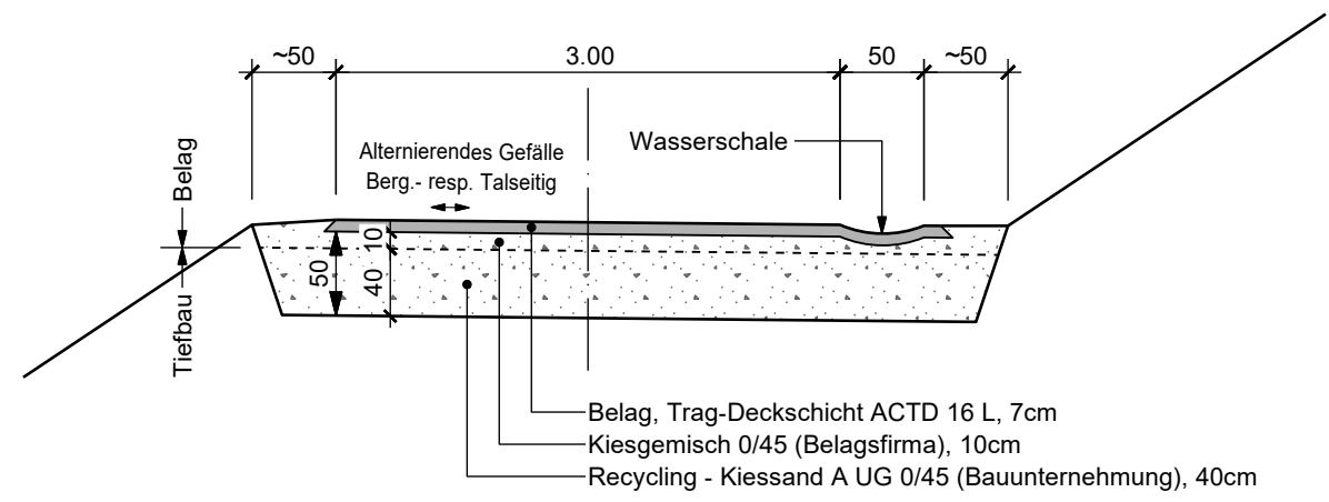
Normalprofil 1:50
